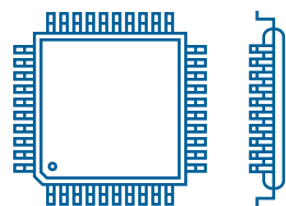
TQFP44-EPAD (10 mm × 10 mm)
