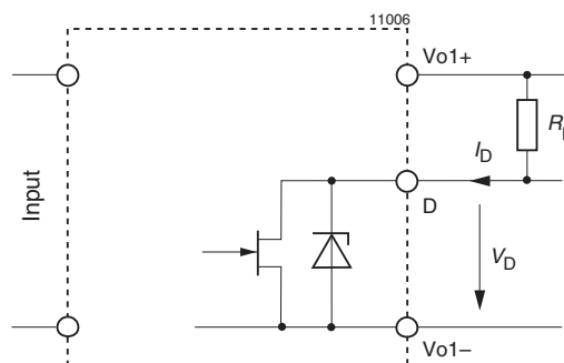
Fig. 15 Options D1 to D4, JFET output
