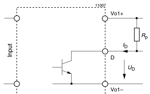
Fig. 16 Options D5...D8, NPN output
