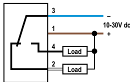
NPN
