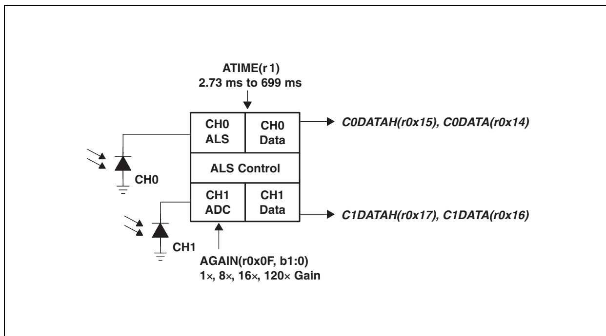
Figure 22: ALS Operation
