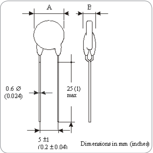
Type YQ Dimensions
