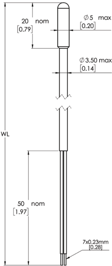
NTC Type JI - Dimensions
