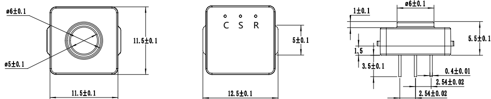
PS1-H2S-5000
