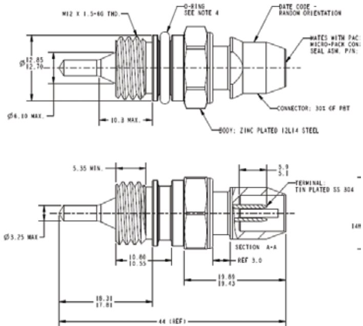
GE-1920 Dimensions
